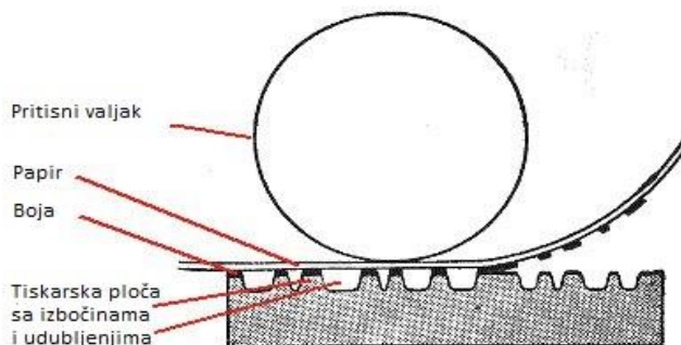
Slika 1. Prikaz visokog tiska
