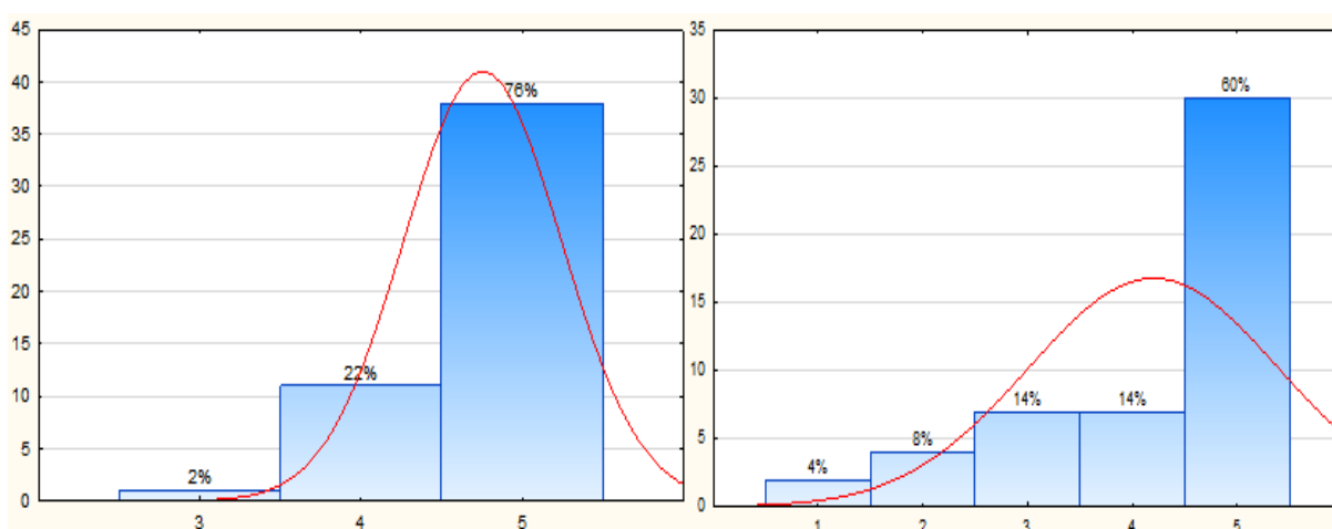
Graf 8. Histogramm der Frequenz für die Variable KAOG Graf 9. Histogramm der Frequenz für die Variable KAOK
