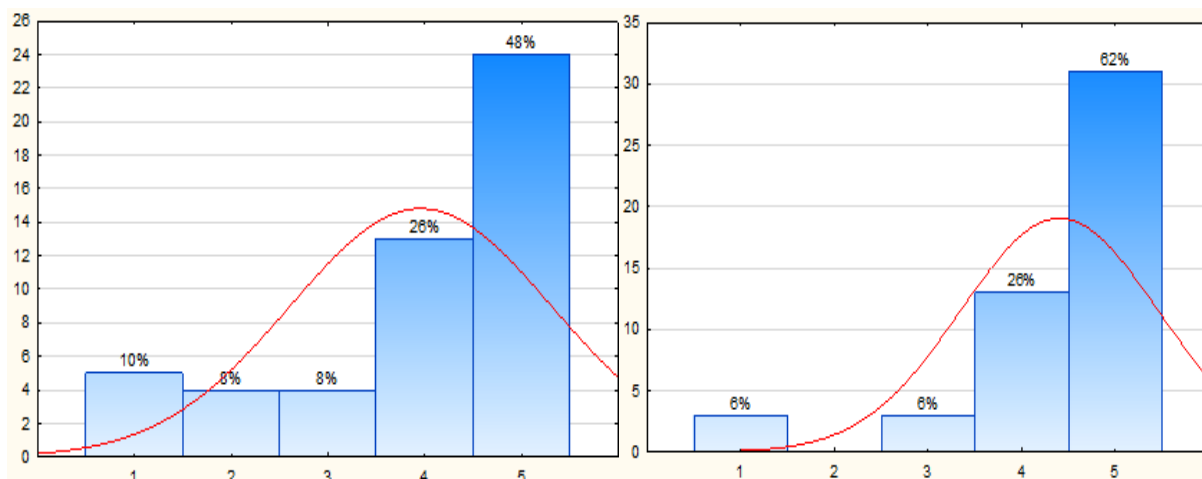
Graf 6. Histogramm der Frequenz für die Variable KAOS Graf 7. Histogramm der Frequenz für die Variable KAOB
