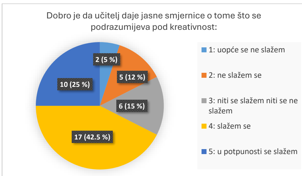
Graf 4: 7. tvrdnja
