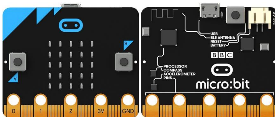
Slika 32. Izgled prednje i stražnje strane BBC micro:bit-a (Preuzeto: 17.3.2020 na: https://www.vidi.hr/Racunala/Novosti/Bakic-oprema-500-skola-BBC-Micro-Bit-racunalima )
