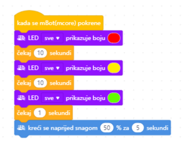
Slika 28. Program semafora
