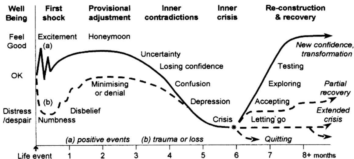
Slika 8. Krivulja učenja
