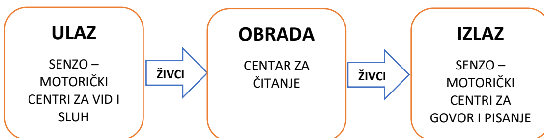
Slika 1: Proces obrade podataka u mozgu prilikom čitanja, izvor: obrada autora prema Pavličević – Franić (2005) i Merck Sharp i Dohme Dostupno na: http://www.msdpriprucnici.placebo.hr/msd-za-pacijente/bolesti-mozga-i-zivcanog-sustava/biologija-zivcanog-sustava/mozak [Pristupljeno 28. studenoga 2017.]
