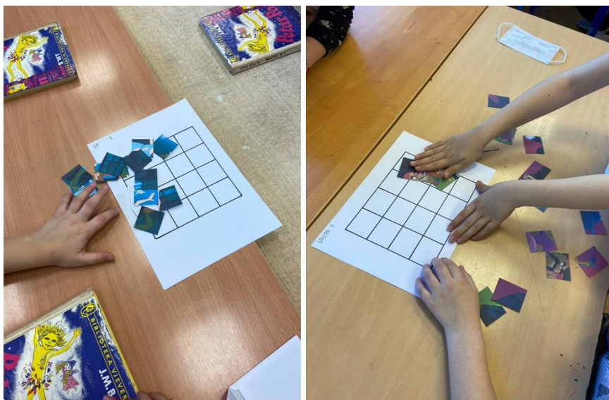
Slika 2. Slaganje slagalice
