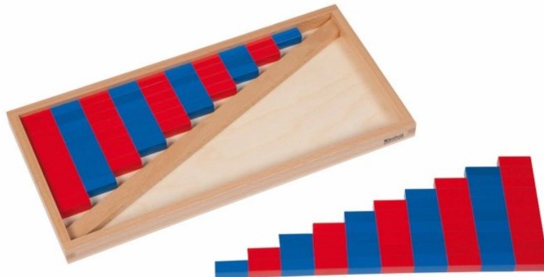
Slika 15. Brojevni prutovi
