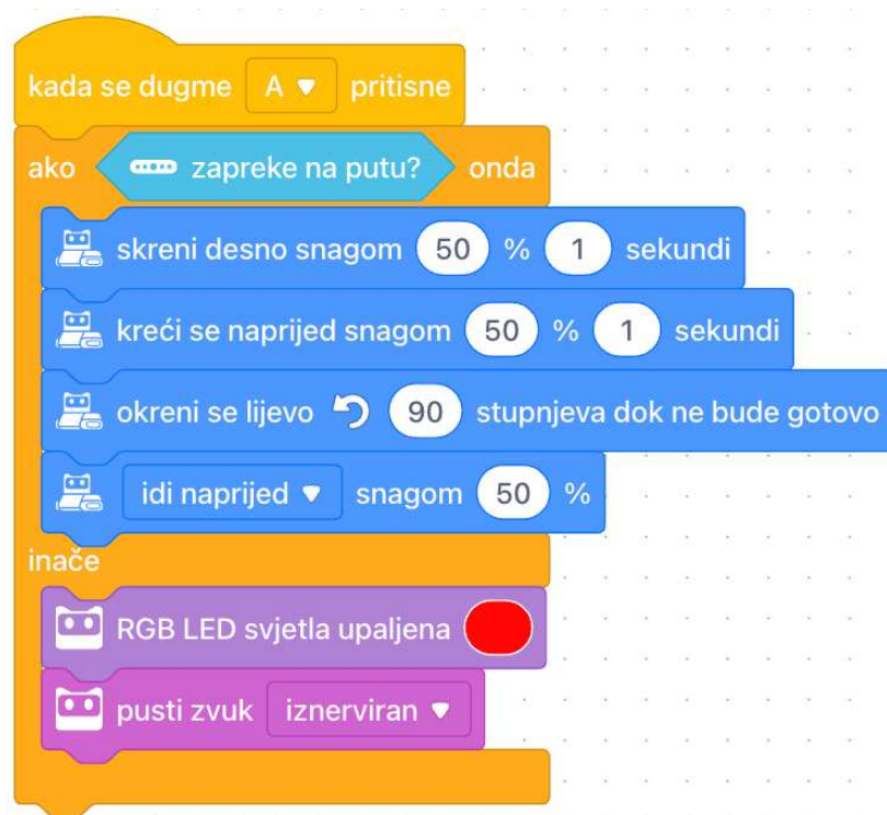
Slika 24. Prošireni program u kojem se koristi uvjetna naredba s „inače“, grananje
